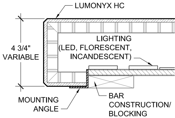
BAR TOP DETAIL A SCALE: 3" = 1'
